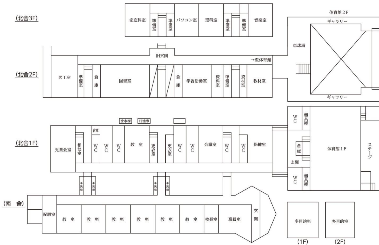
牧田小学校跡地施設校舎等平面図
